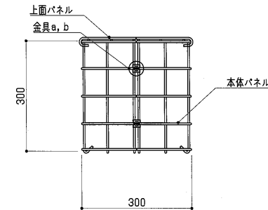
側面図 S=1:10
