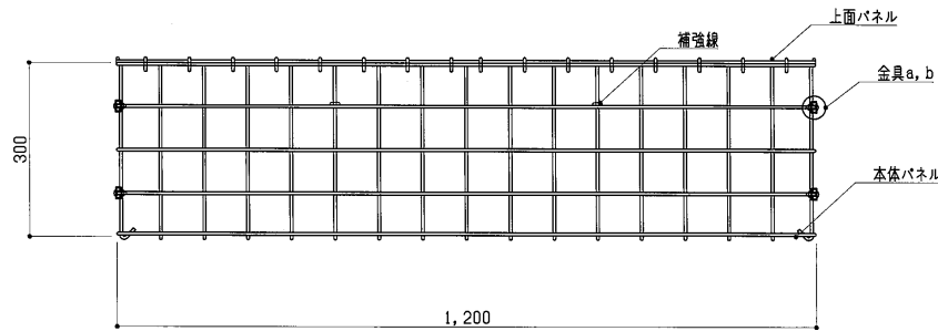
正面図 S=1:10
