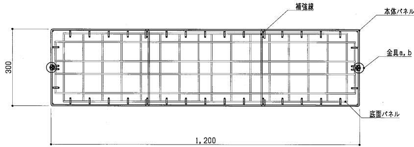
断面図 S=1:10
