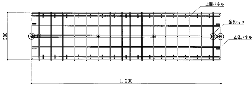
平面図 S=1:10
